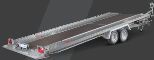
ATH 27-49-21.2 mit Boden
